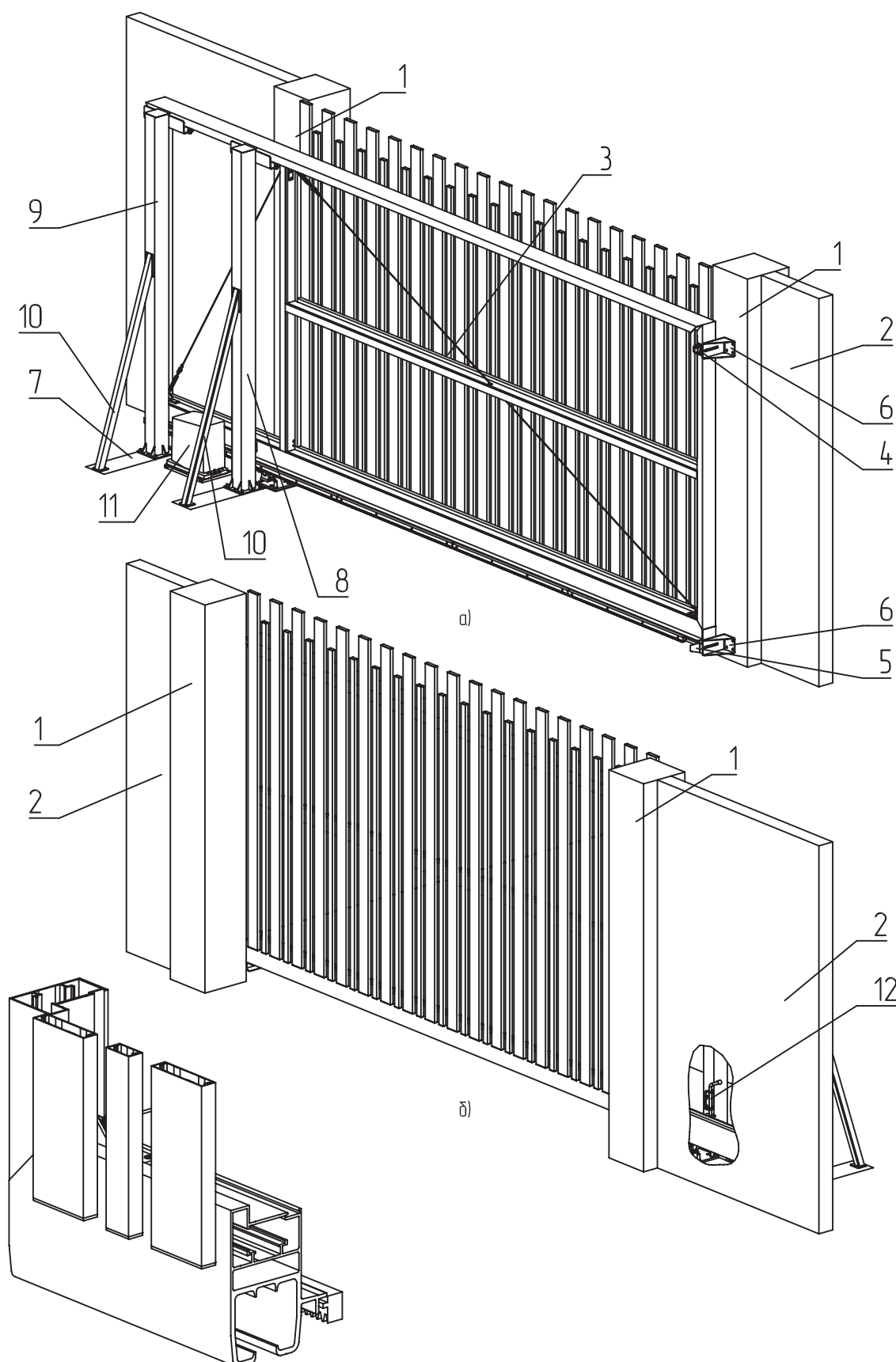
Рисунок 7.6. Откатные самонесущие ворота с накладным вертикальным разреженным заполнением алюминиевыми профилями, открытие влево
