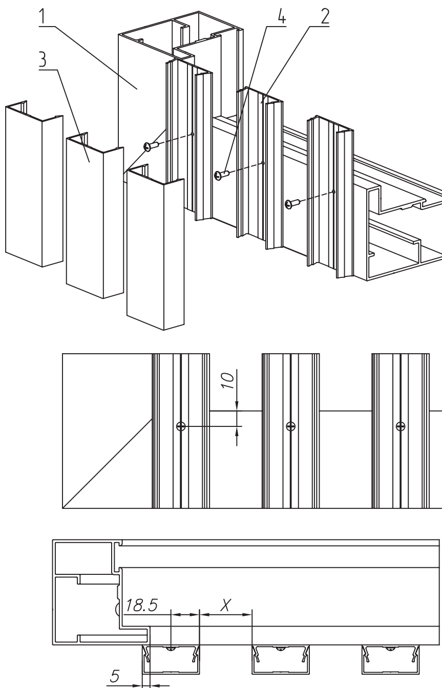
Рисунок 8.7 Монтаж заполнения с накладным типом монтажа из профилей разреженного заполнения шириной 37 мм 1 – створка, 2 – профиль монтажный FLGU.400.0402, 3 – профиль разреженного заполнения FLGU.400.0404, 4 – винт самонарезающий 3,5x9,5SAX.
