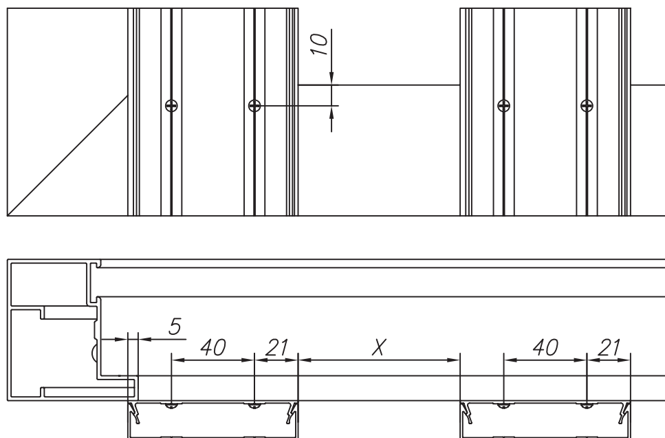
Рисунок 8.6 Монтаж заполнения с накладным типом монтажа из профилей разреженного заполнения шириной 82 мм 1 – створка, 2 – профиль монтажный FLGU.400.0401, 3 – профиль разреженного заполнения FLGU.400.0403, 4 – винт самонарезающий 3,5x9,5SAX.
