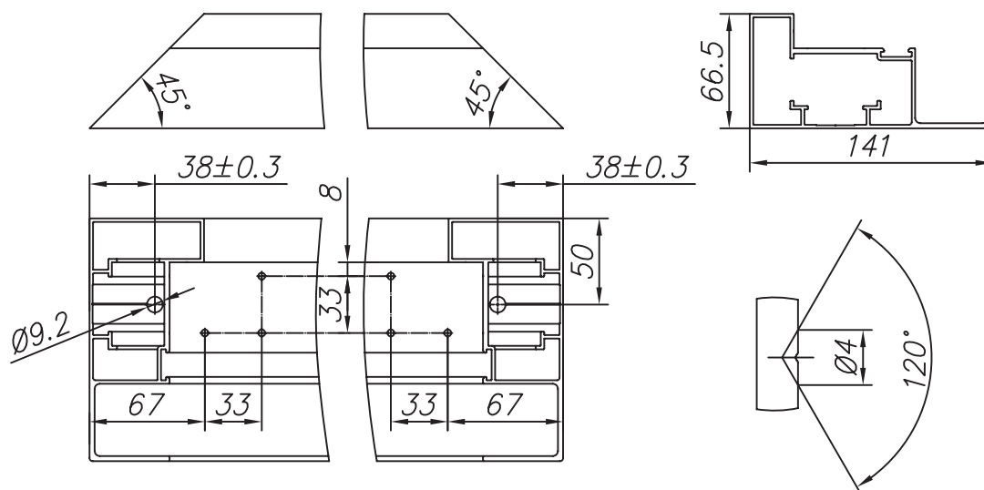
Рисунок 10.4 Изготовление балки
