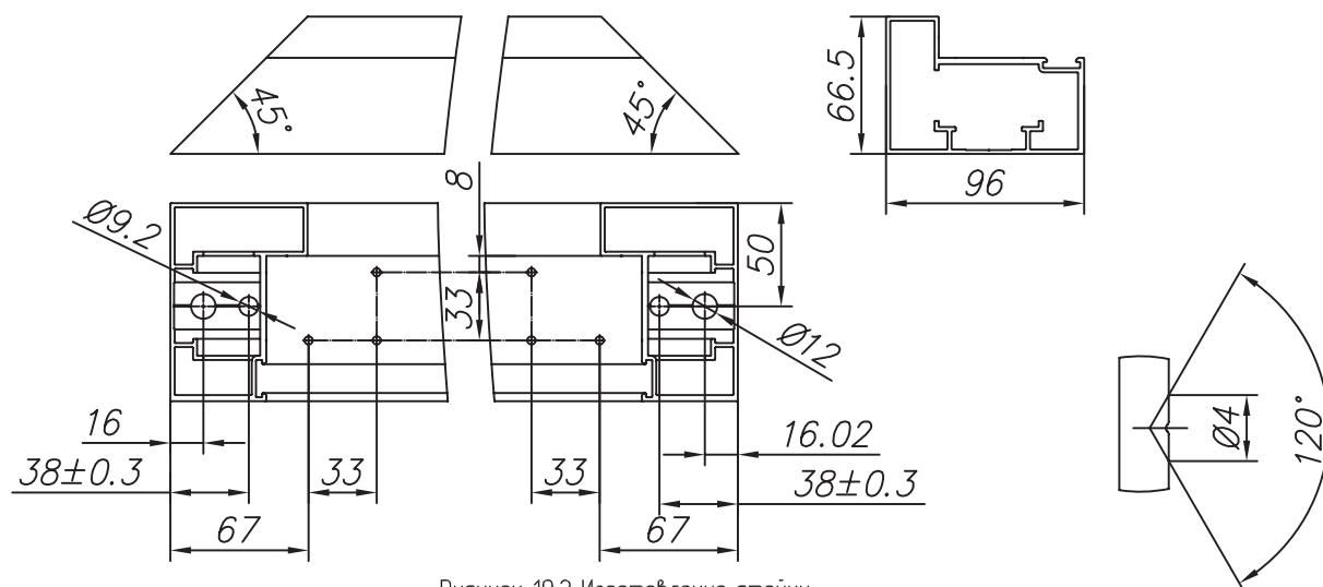
Рисунок 10.2 Изготовление стойки
