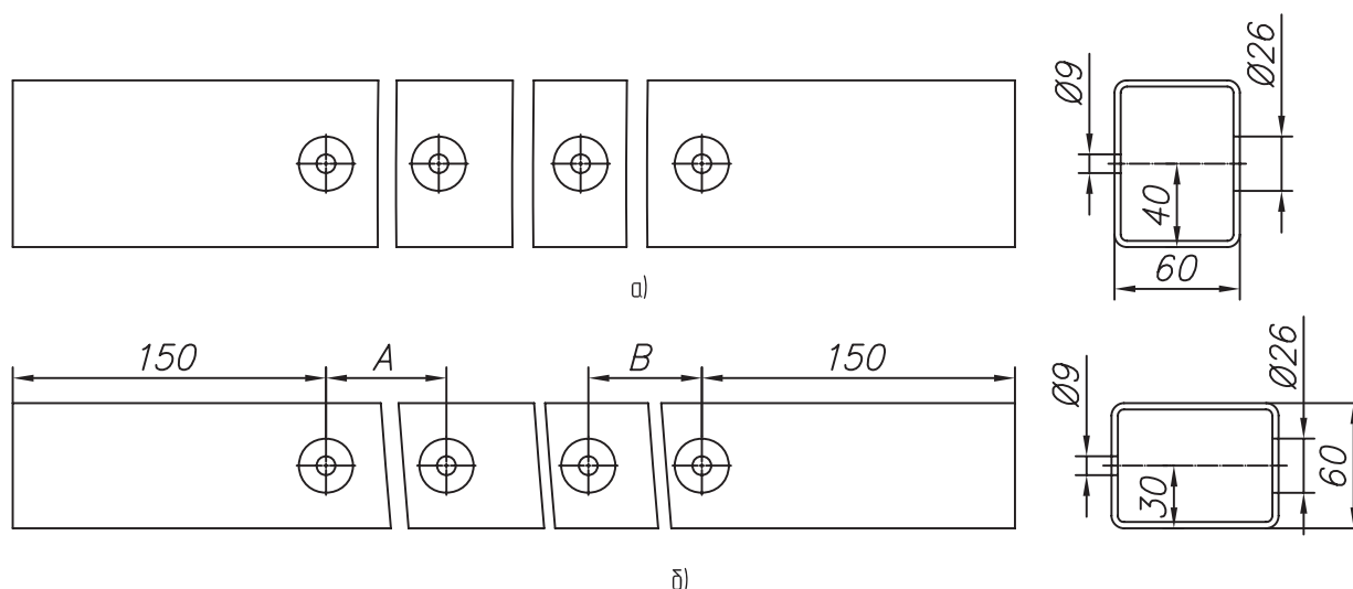
Рисунок 10.12 Изготовление столба створки распашных ворот а – при встроеном монтаже ворот, б – при накладном монтаже
