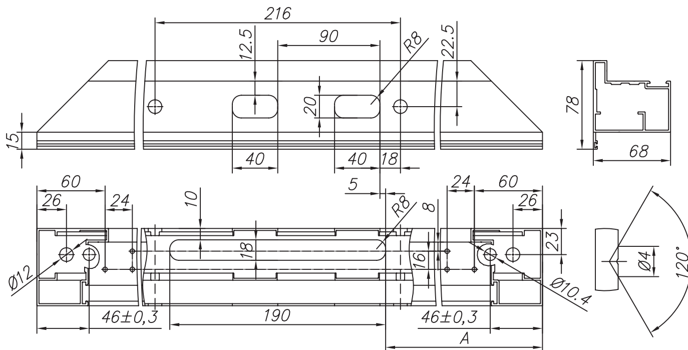
Рисунок 10.26 Изготовление стойки с пазом для замка из профиля FLGU.400.0108 (открытие наружу, влево) На нижнем виде показано сечение по оси отверстия \varnothing 12 мм
