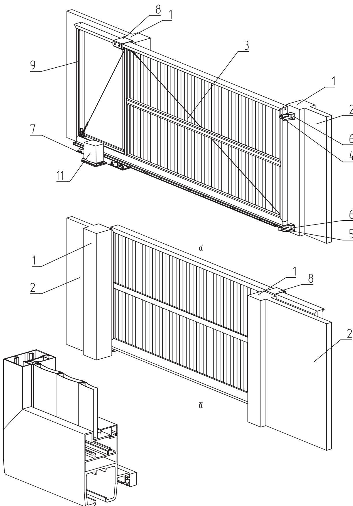
Рисунок 7.8. Откатные самонесущие ворота с вертикальным заполнением из профиля AG77, открывание влево, без столбов удерживающих
