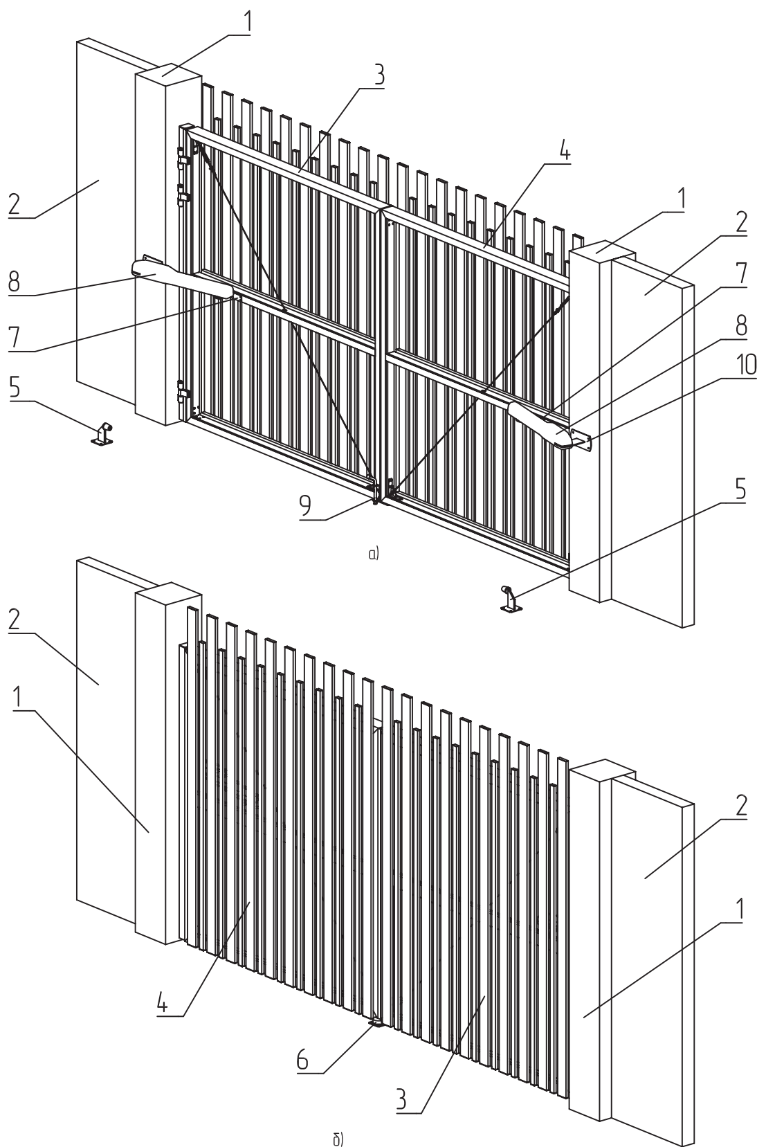
Рисунок 7.11. Распашные ворота со встроенным типом монтажа, открывание внутрь с накладным вертикальным закрепом алюминиевыми профилями а – вид со стороны двора, б – вид со стороны улицы 1 – столб проема, 2 – забор, 3 – створка ворот с заполнением левая, 4 – створка ворот с заполнением правая, 5 – упор боковой, 6 – упор центральный, 7 – кронштейн для крепления электропривода к створке, 8 – электропривод, 9 – засов, 10 – кронштейн для крепления электропривода к столбу проема.
