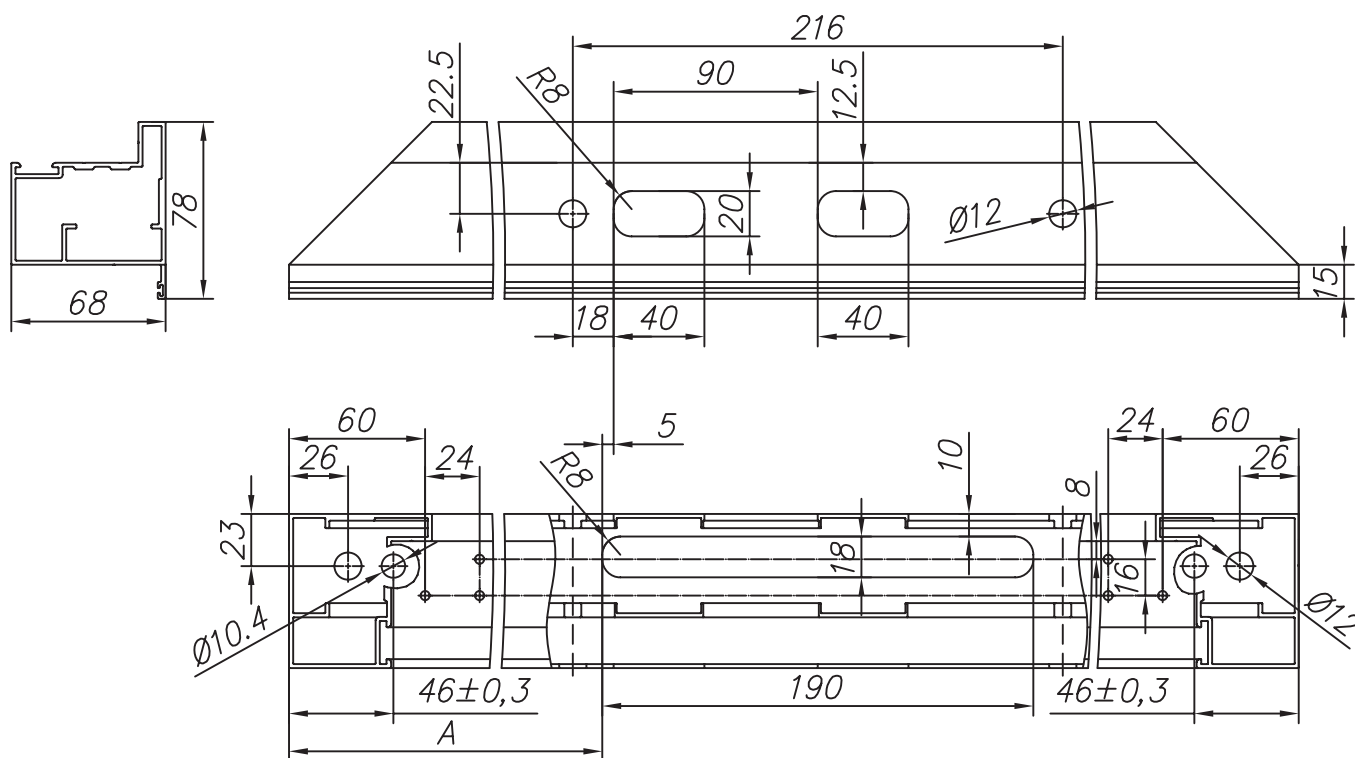
Рисунок 10.27 Изготовление стойки с пазом для замка из профиля FLGU.400.0108 (открытие наружу, вправо) На нижнем виде показано сечение по оси отверстия \varnothing 12 мм
