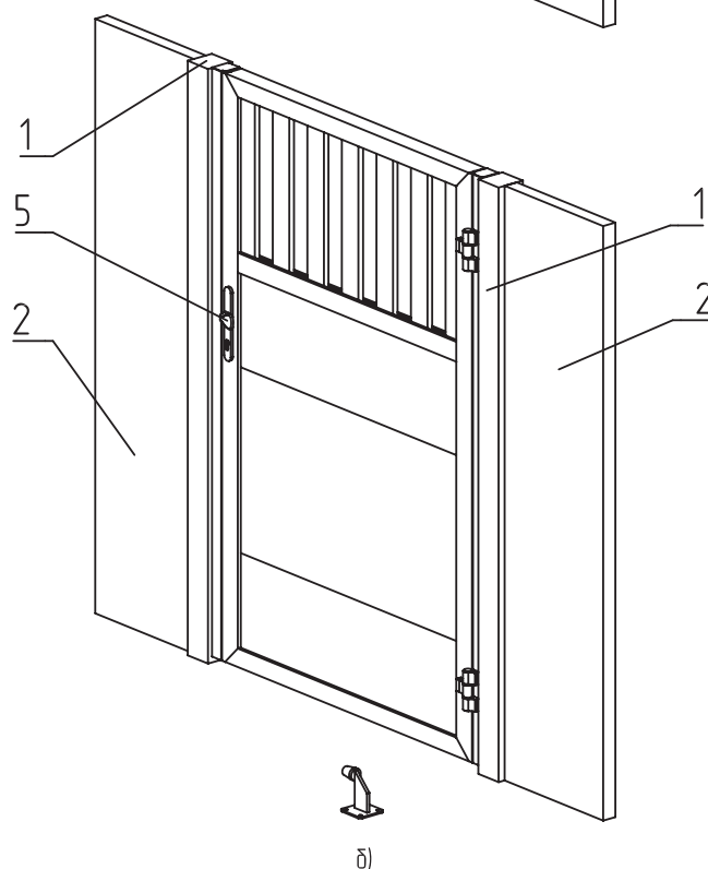
Рисунок 7.21. Калитка со встроенным монтажем, направлением открывания вправо, наружу с комбинированным заполнением из сэндвич-панели и алюминиевого профиля
