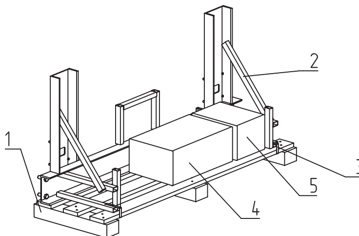
Рисунок 11.8 Упаковка рамы ворот опорной и коробок с комплектацией (FLGU.400.9801-03) 1 – поддон FLGU.400.9904, 2 – рама ворот опорная, 3 – лента полипропиленовая, 4 – коробка (lxbxh=510x310x200, 5 – коробка с опорами роликовыми (lxbxh=320x240x200)
