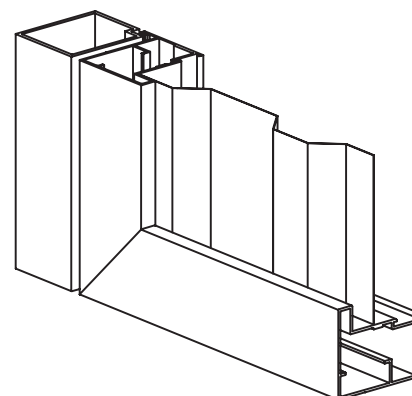
Рисунок 7.20. Калитка со встроенным монтажом, направлением открывания влево, наружу с вертикальным встроенным заполнением из профилированного листа
