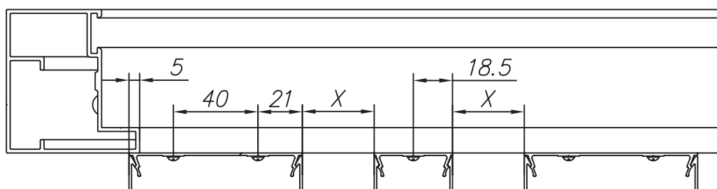
Рисунок 8.8 Монтаж разреженного заполнения с накладным типом монтажа из сочетания профилей заполнения шириной 82 мм и 37 мм 1 – створка, 2 – профиль монтажный FLGU.400.0401, 3 – профиль монтажный FLGU.400.0402, 4 – профиль разреженного заполнения FLGU.400.0403, 5 – профиль разреженного заполнения FLGU.400.0404, 6 – винт самонарезающий 3,5х9,5SAX.
