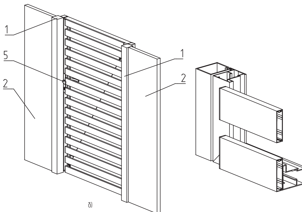
Рисунок 7.17. Калитка с накладным монтажом, направлением открывания влево, внутрь с горизонтальным накладным разрезным заполнением алюминиевыми профилями а – вид со стороны двора, б – вид со стороны улицы
