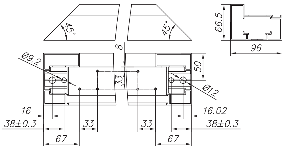
Рисунок 10.14 Изготовление стойки (профиль рамы FLGU.400.0102)
