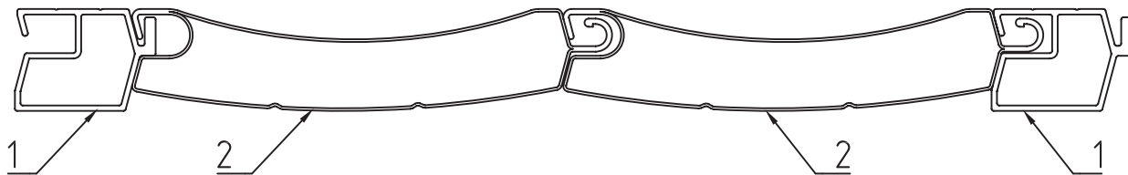
Рисунок 8.20 Заполнение AG/77 1 – профиль притвора 400.0501, 2 – профиль AG/77
