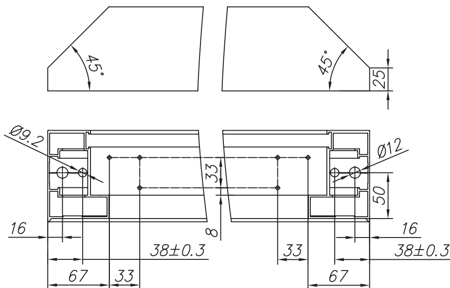
Рисунок 10.15 Изготовление стойки (профиль рамы FLGU.400.0105)
