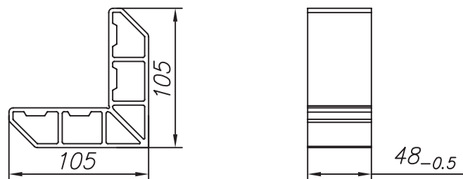
Рисунок 10.7 Изготовление соединителя углового FLGU.400.0910
