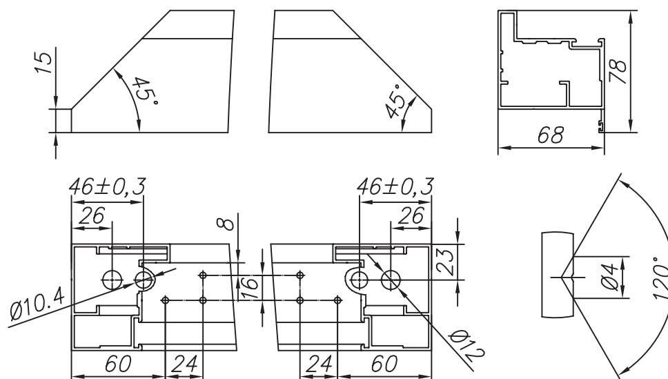
Рисунок 10.28 Изготовление стойки без паза для замка из профиля FLGU.400.0110 (открытие внутрь)
