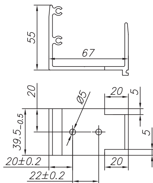
Рисунок 10.9 Изготовление соединителя FLGU.400.0912
