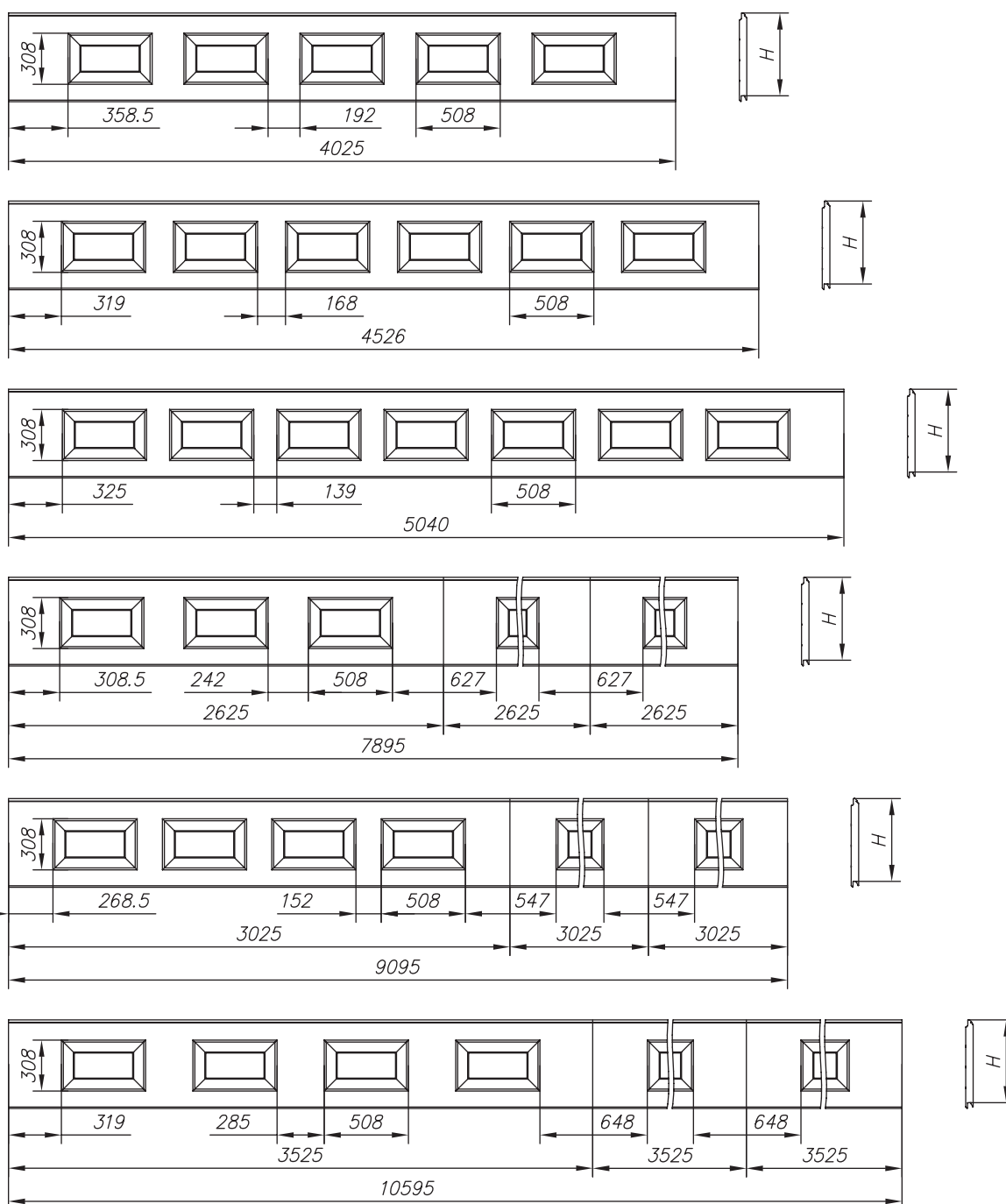
Рисунок 3.3 Схематическое изображение сэндвич-панели с рисунком «филенка»
