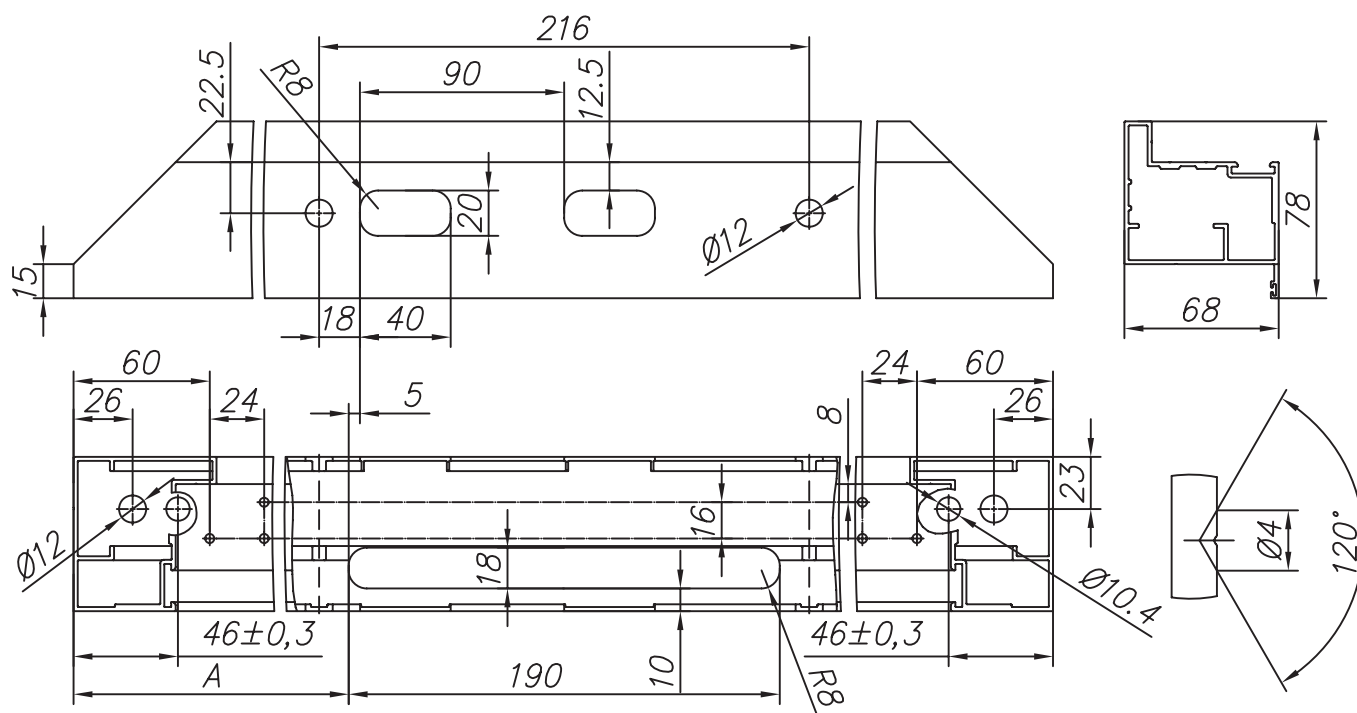
Рисунок 10.28 Изготовление стойки без паза для замка из профиля FLGU.400.0110 (открытие внутрь)
