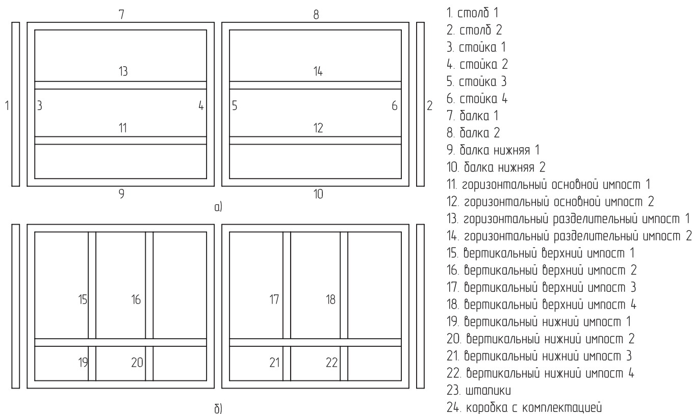
Рисунок 11.21 Схематическое изображение распашных ворот с максимальным количеством деталей
