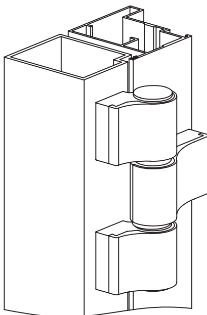
Направления регулировки петли FLGU.400.1002
