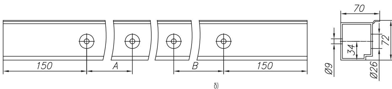
Рисунок 10.35 Изготовление столба FLGU.400.0502 при встроеном монтаже калитки (открывание внутрь, наружу)
