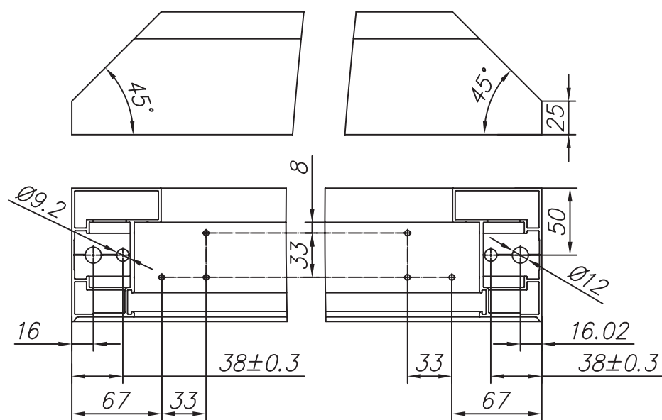
Рисунок 10.16 Изготовление стойки (профиль рамы FLGU.400.0106)
