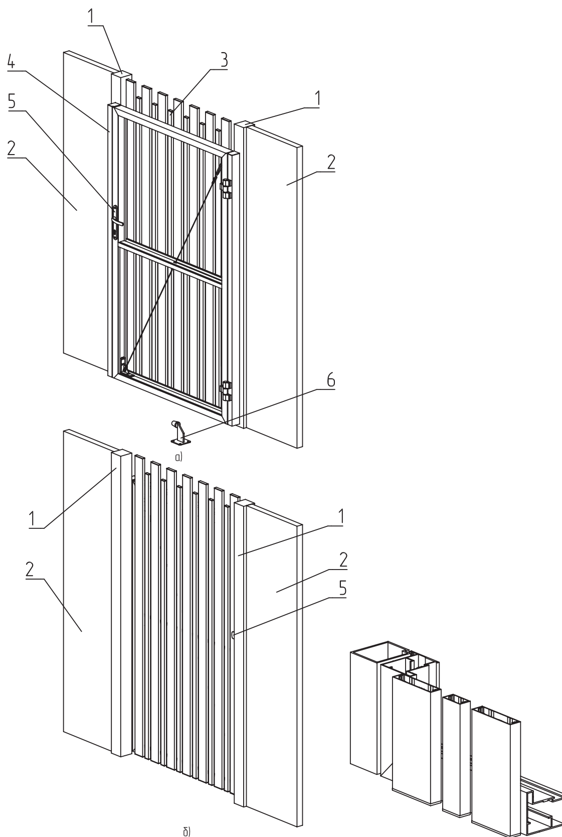
Рисунок 7.18. Калитка с накладным монтажом, направлением открывания вправо, внутрь с вертикальным накладным разрезным заполнением алюминиевыми профилями (гребенка)
