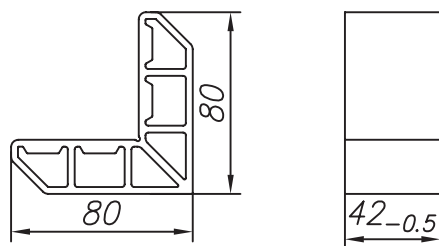
Рисунок 10.34 Изготовление соединителя углового FLGU.400.0914
