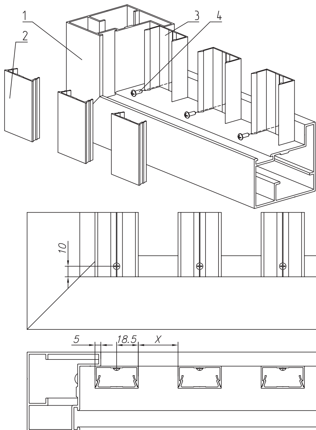
Рисунок 8.3 Монтаж заполнения со встроенным типом монтажа из профиля разреженного заполнения шириной 37 мм 1 – створка, 2 – профиль монтажный FLGU.400.0402, 3 – профиль разреженного заполнения FLGU.400.0404, 4 – винт самонарезающий 3,5x9,5SAX.
