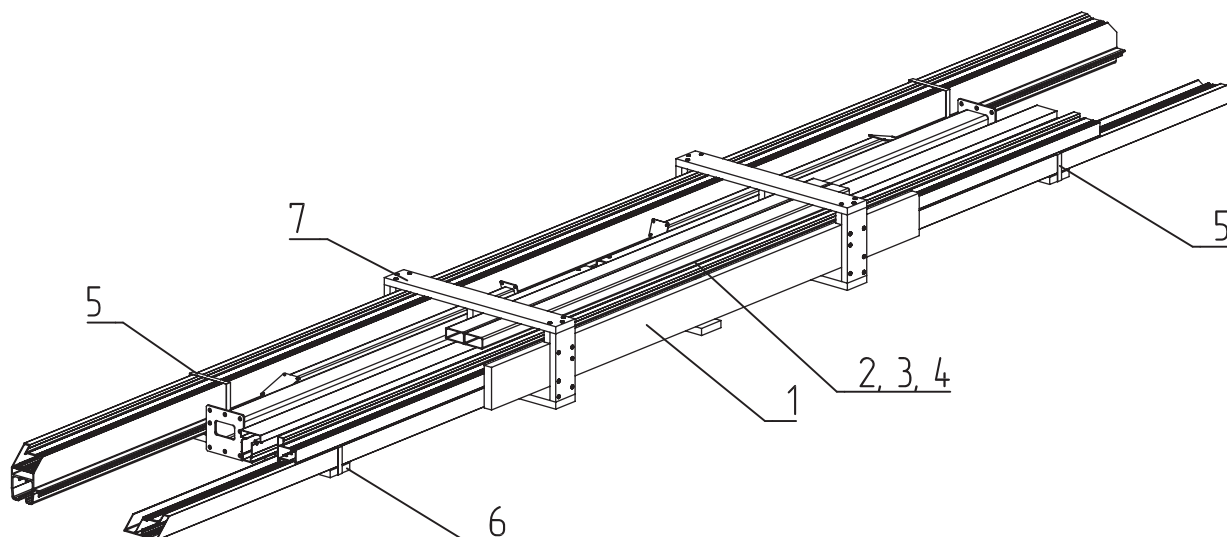
Рисунок 11.7 Упаковка деталей рамы откатных ворот, столбов, раскосов (FLGU.400.9801-01) 1 – поддон FLGU.400.9902, 2 – детали рамы, 3 – столбы, раскосы, 4 – профили заполнения, 5 – лента полипропиленовая, 6 – доска поддерживающая (FLGU.400.9902.07), 7 – доска поддона (FLGU.400.9902.01)
